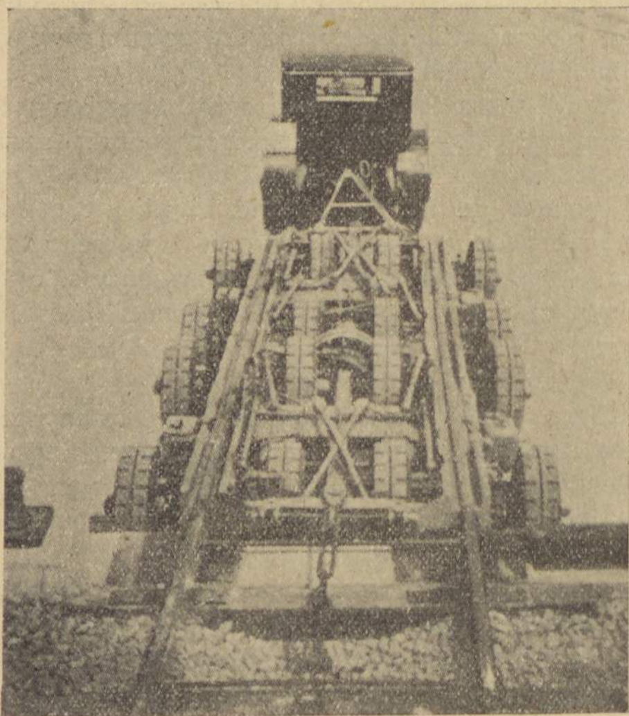
Esta gravura mostra dois grandes «bogies» com o camion, no cais pronto a receber o vagon de mercadorias. Nesta gravura vêem-se perfeitamente os varões para ajuntamento das rodas
