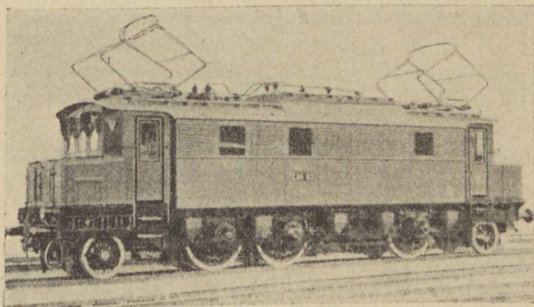
Locomotora A. E. G. capaz de conseguir umr velocidade máxima de 151,5 km. poa hora, atrelada a um comboio expresso completo
