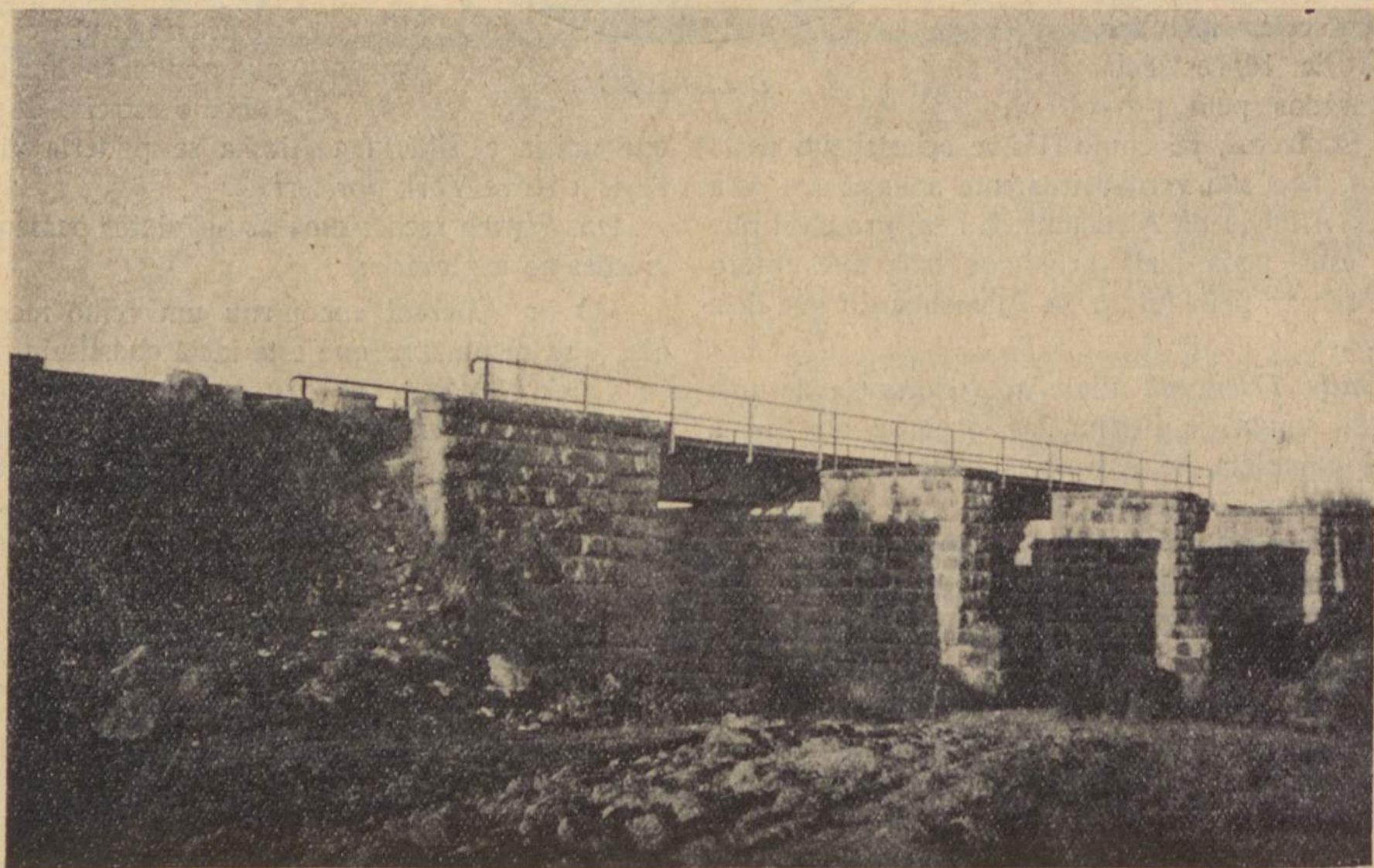
LINHA DE ÉVORA - Pontão ao Km. 97,573,55
