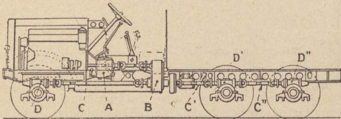
Esquema dum veículo ligeiro para transporte de tropas num terreno variado com 6 rodas independentes e tractores
