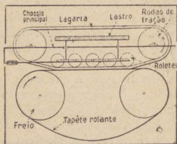
Banco de ensaio para os «lagartas» dos carros de assalto e de tracção destinado a obter dados exactos sobre a resistência e desgaste das suas peças
