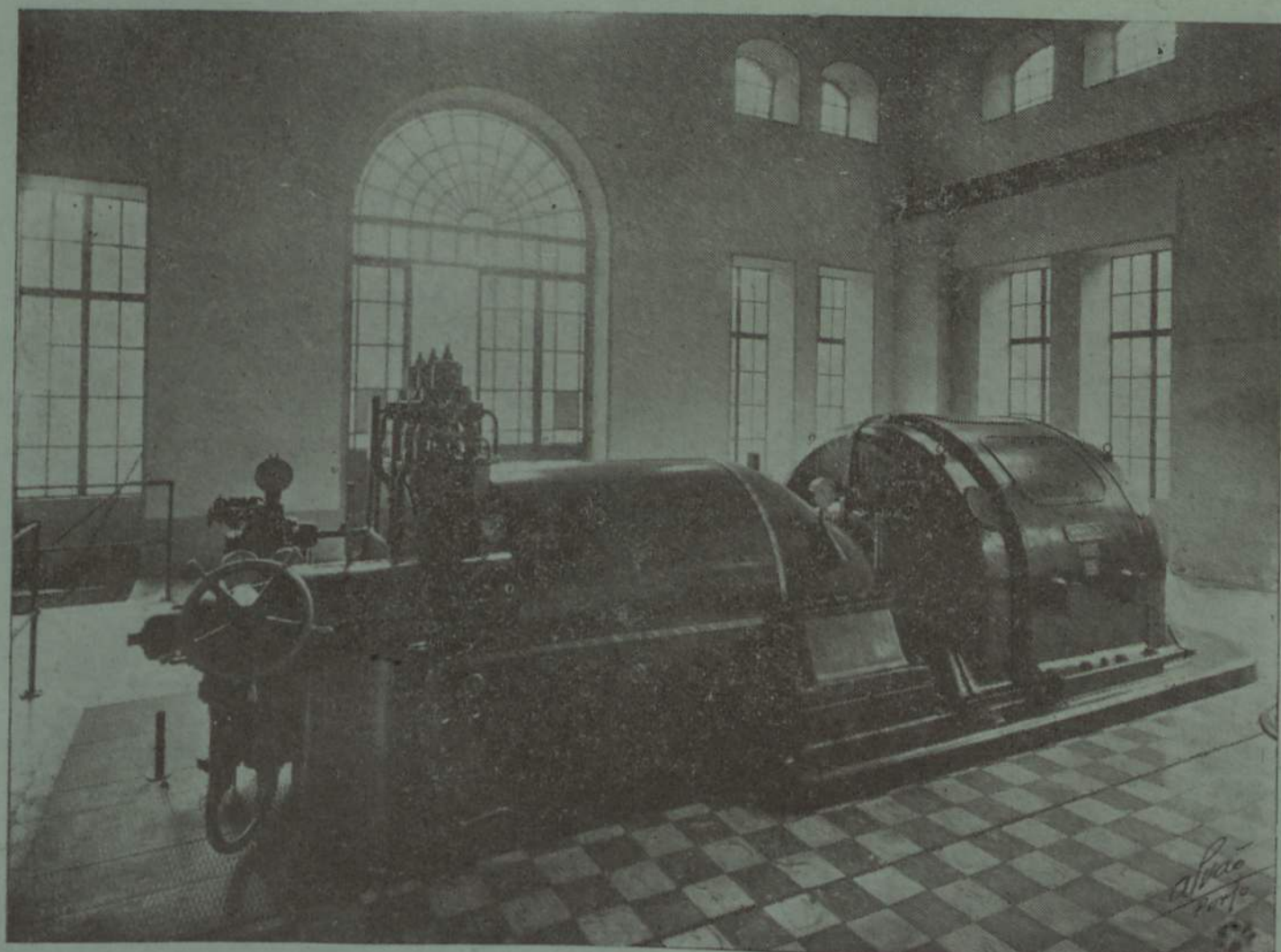
Turbo-grupo a vapor BROWN-BOVERI de 6400 kilowatts na central termica de Caniços da Companhia Hidro-Eléctrica do Varosa
