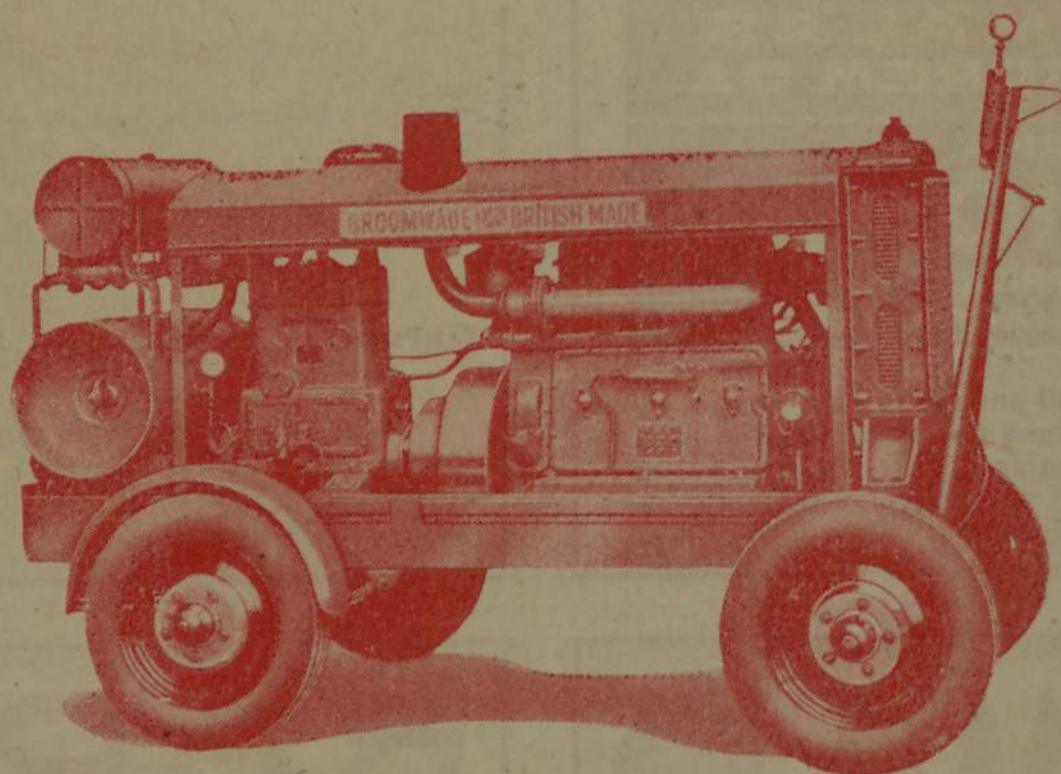
Compressor Transportável Broom Wade
