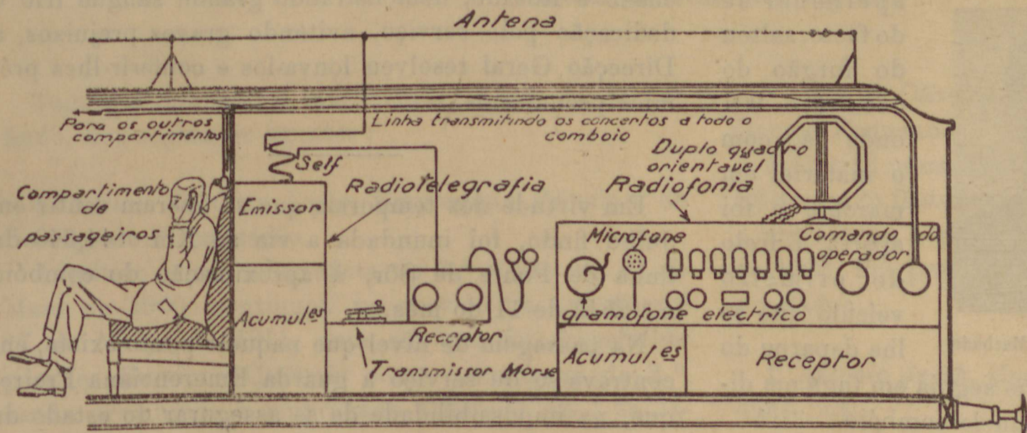
Esquema da instalação radioeléctrica numa carruagem
