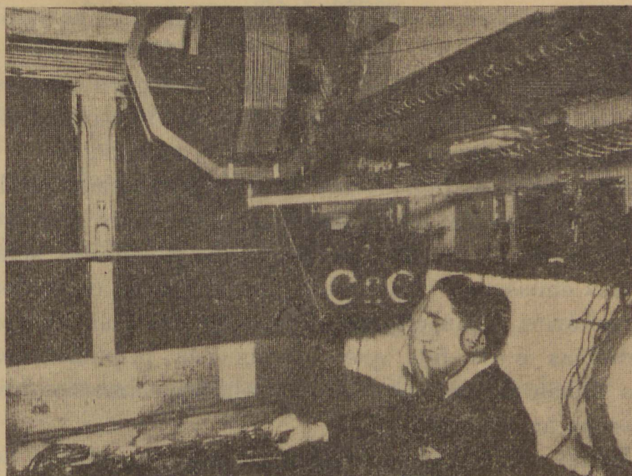
Compartimento onde se encontram instalados os aparelhos. Em cima à direita o quadro para a recepção das emissões radiofônicas; por baixo o aparelho receptor de telegrafia sem fios. O empregado tem na mão o transmissor Morse que está colocado sobre uma caixa que contém o posto receptor de telefonia sem fios; à esquerda o gramofone eléctrico que entra em acção quando falha a transmissão radiofônica.
