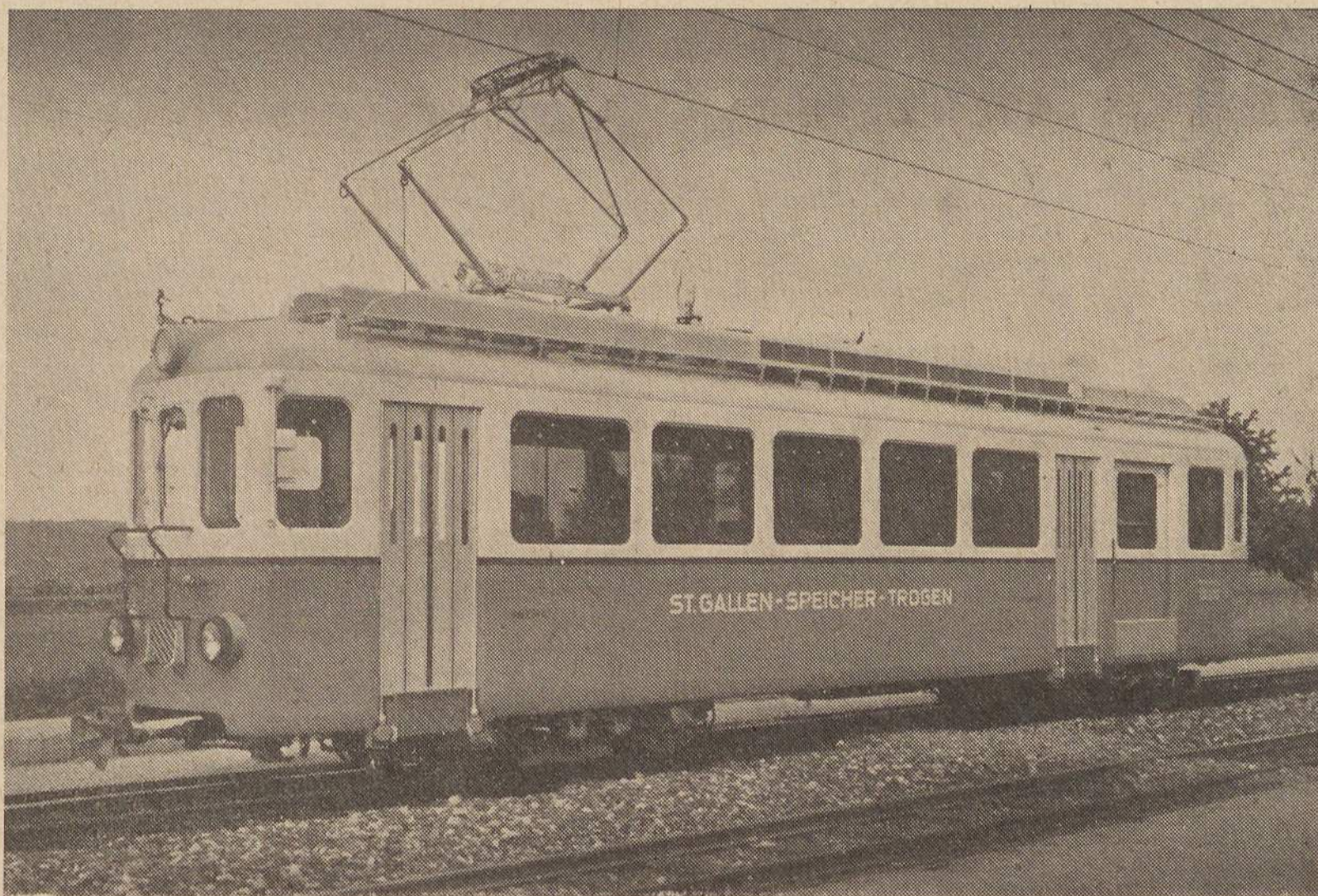
Automotora eléctrica para bitola estreita, com o peso de 27 toneladas, fabricada pela Schindler Wagons S. A.
