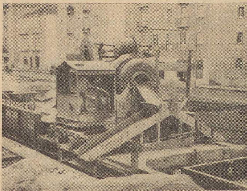
Tipo de betoneira, de um dos comboios de serviço
