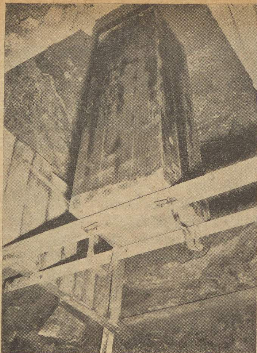
Um furo pronto a ser betonado
