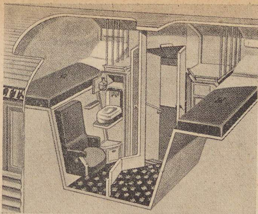
Vista em corte dum grupo de 4 compartimentos
