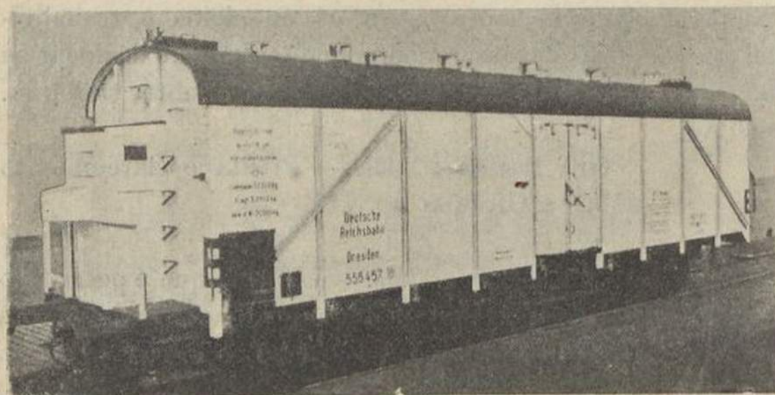
Vagão frigorífico
