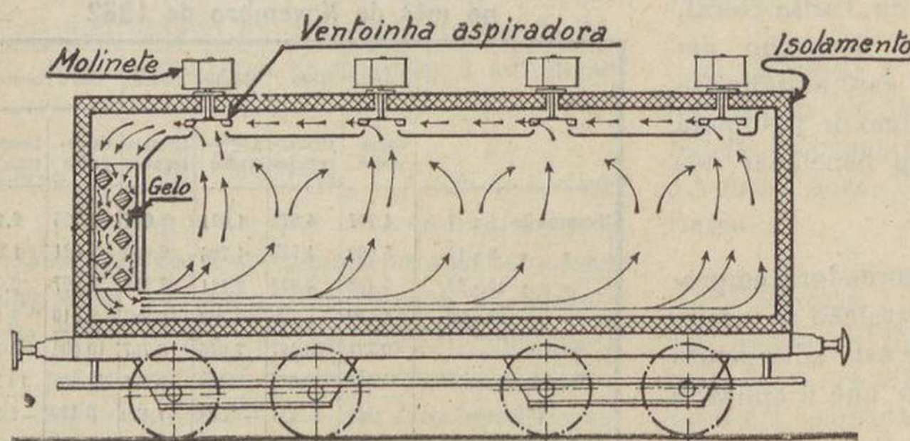
Esquemas do sistema de refrigeração do vagão
