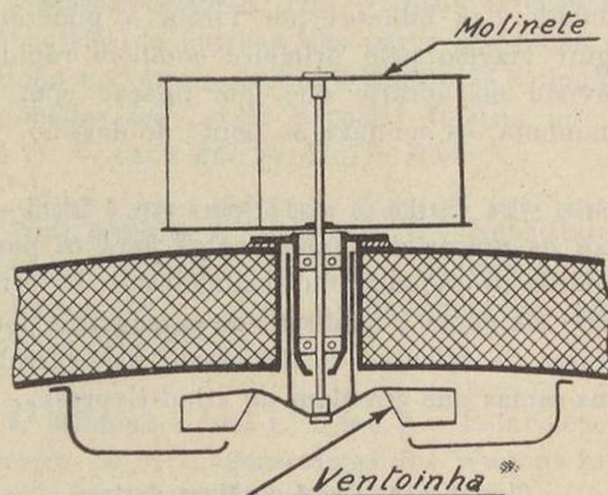
Esquema de uma das ventoinhas
