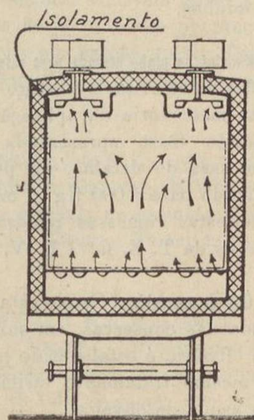
Esquemas do sistema de refrigeração do vagão
