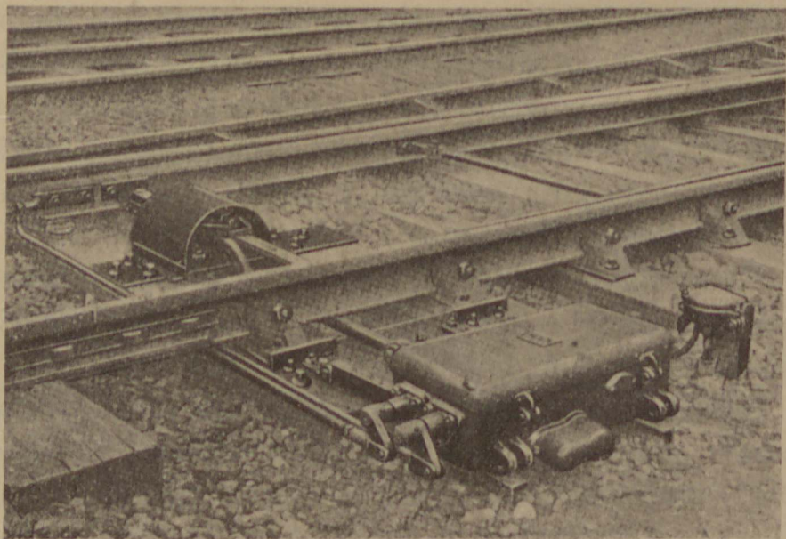
Fig. 2 — Motor de manobra de agulha
