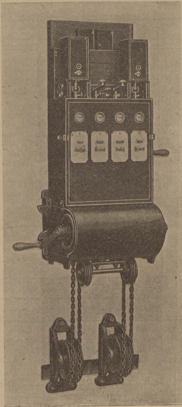
Fig. 3 — Aparelho de bloco manual
